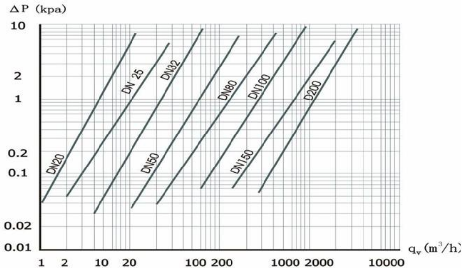
压力损失曲线
